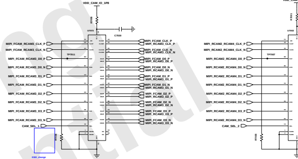
MIPI SWITCH (FCAM,RCAM3)
